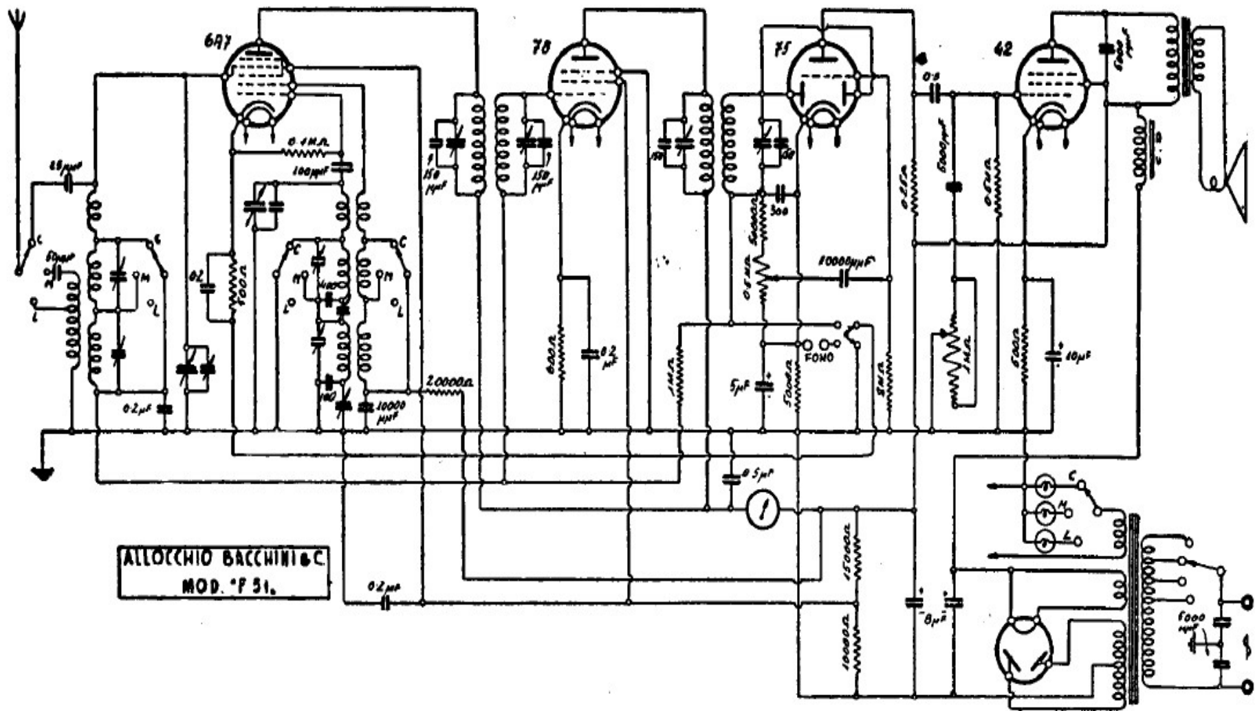
ALLOCCIO, BACCHINI e Co. — Mod. 51 F.M. e Mod 51 G Produzione 1936. • Media freq.: 425 kc.
